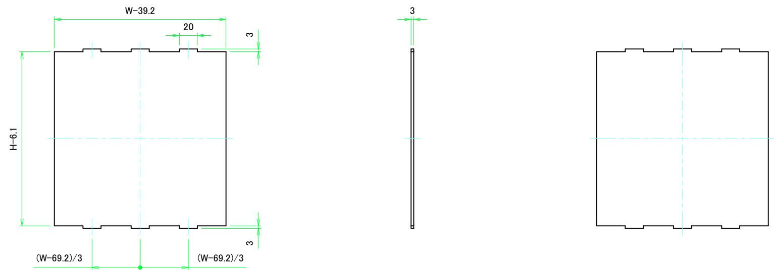
Wパネル1表面 / W Panel 1 Frontside
