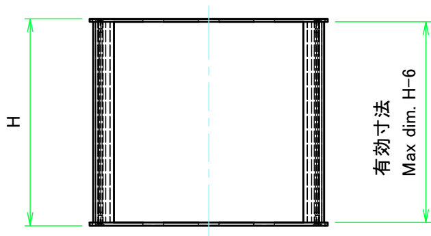
Wパネル1 / W Panel 1
