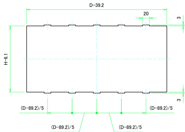
Dパネル1表面 / D Panel 1 Frontside
